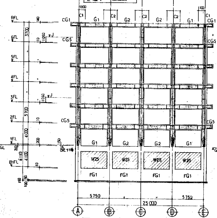
3通り 軸組図
