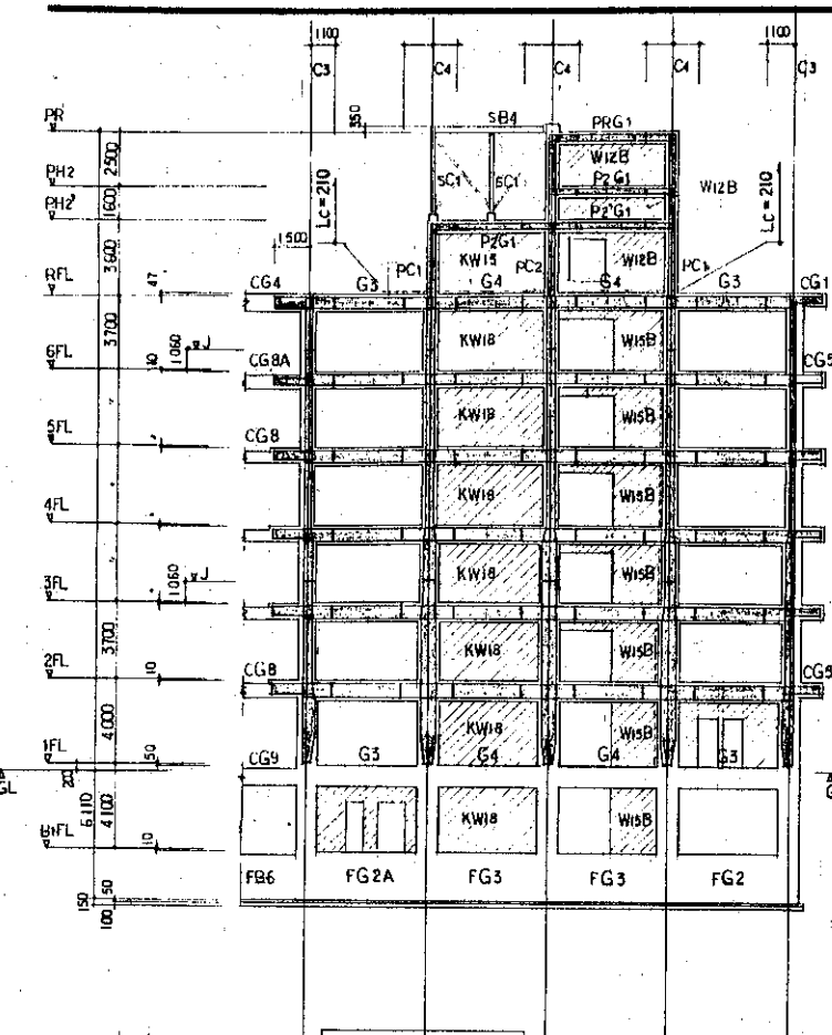
2通り 軸組図
