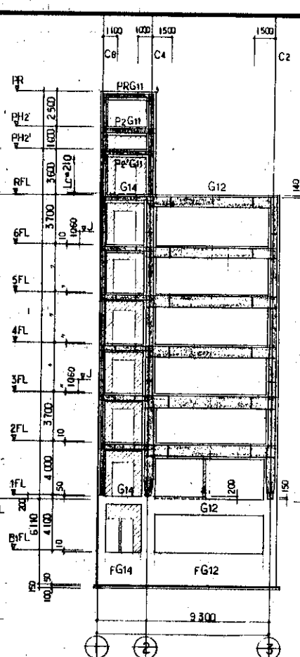
C通り 軸組図
