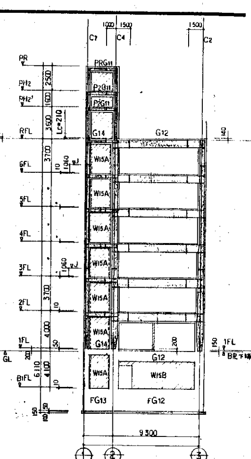
D通り 軸組図
