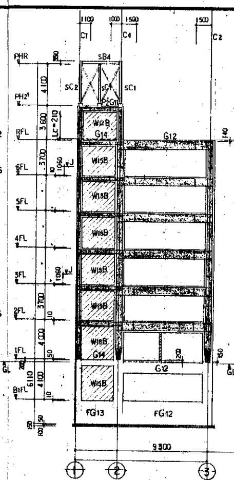
B通り 軸組図
