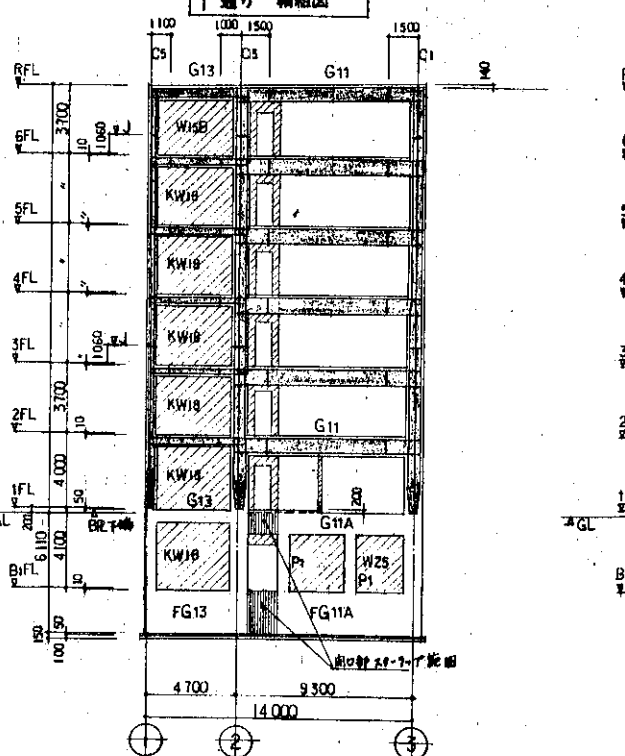
A通り 軸組図
