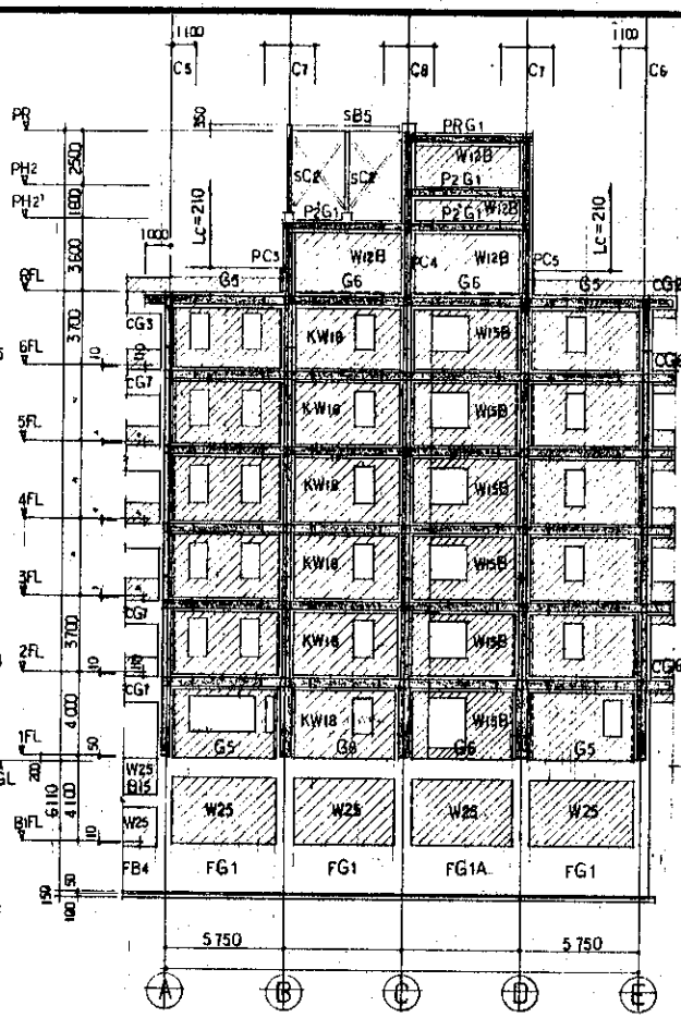
1通り 軸組図
