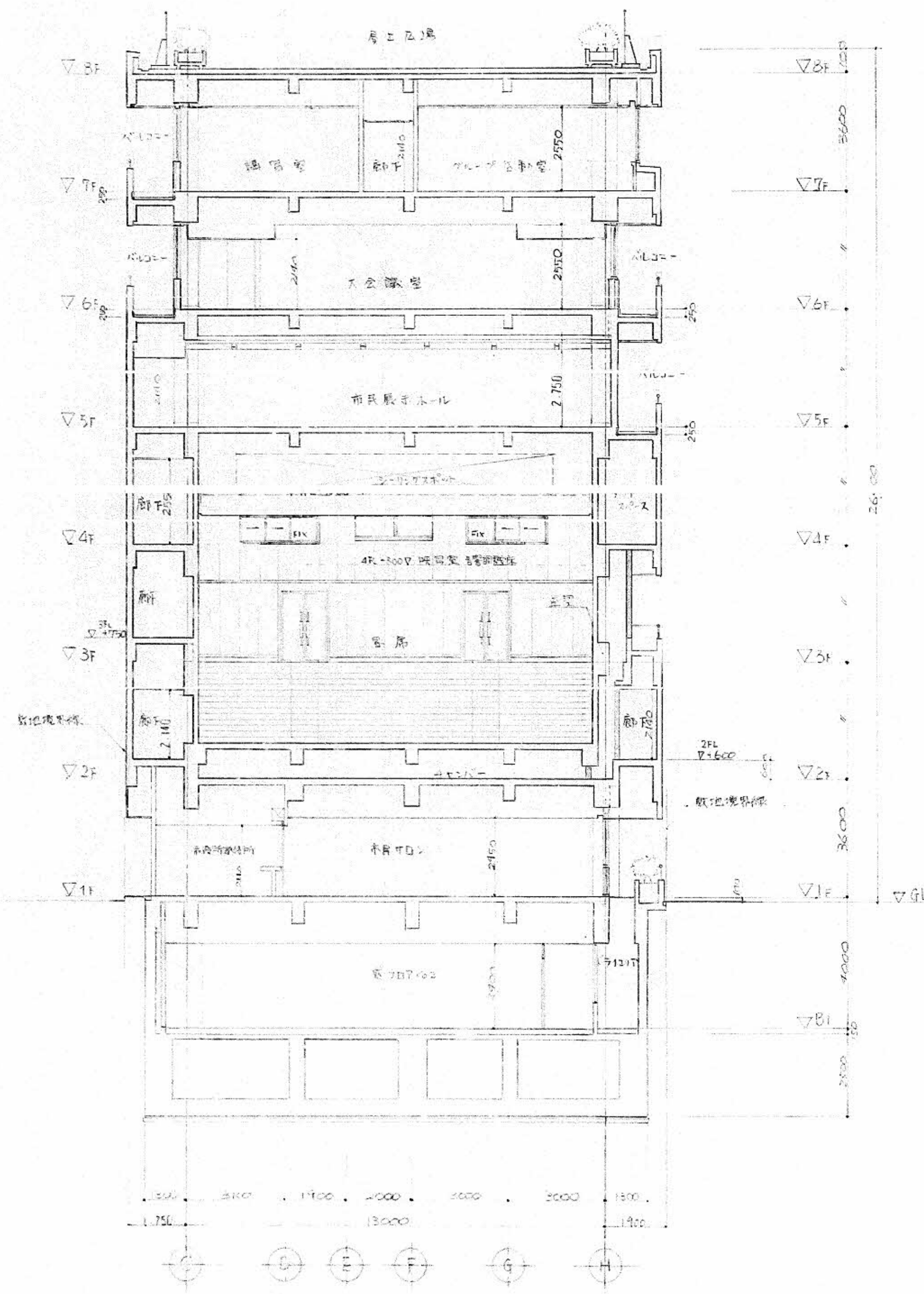
8~9間 断面図
