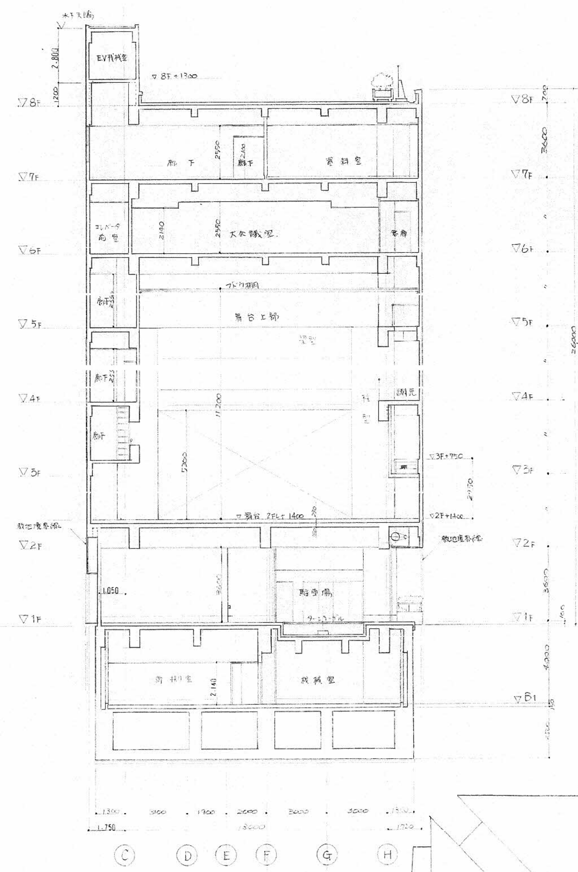
10~11間 断面図
