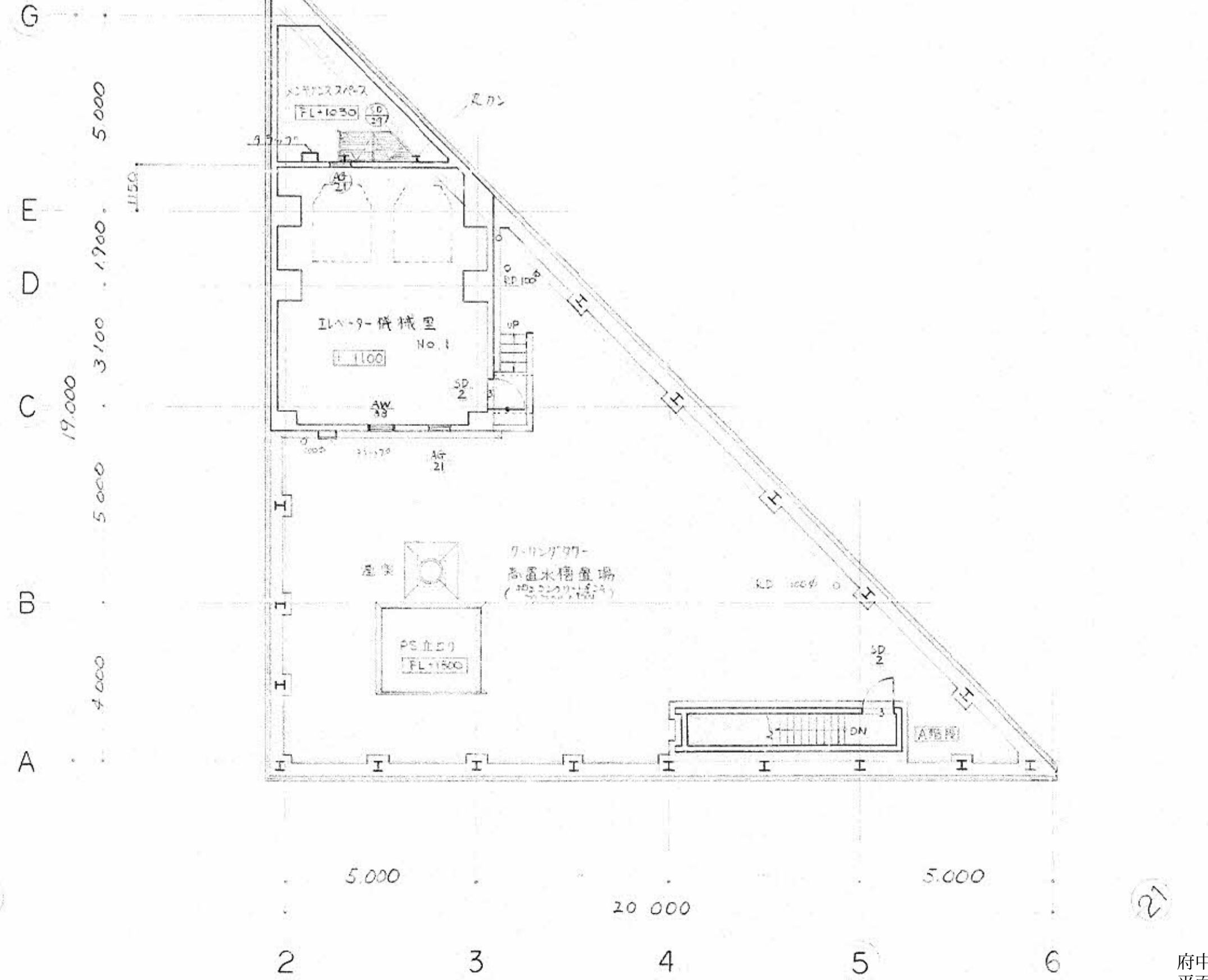
塔屋3階平面図
