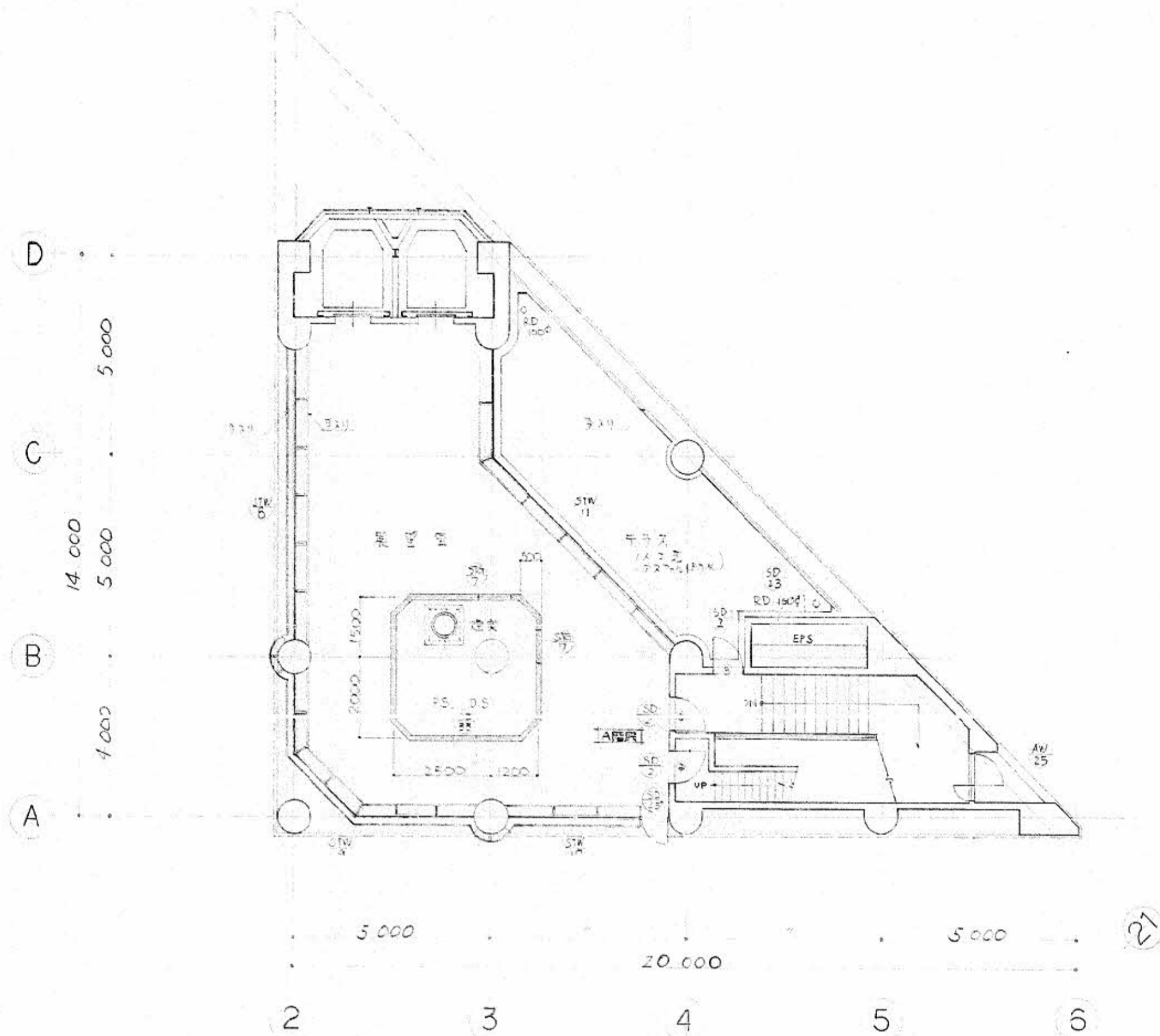
塔屋2階平面図
