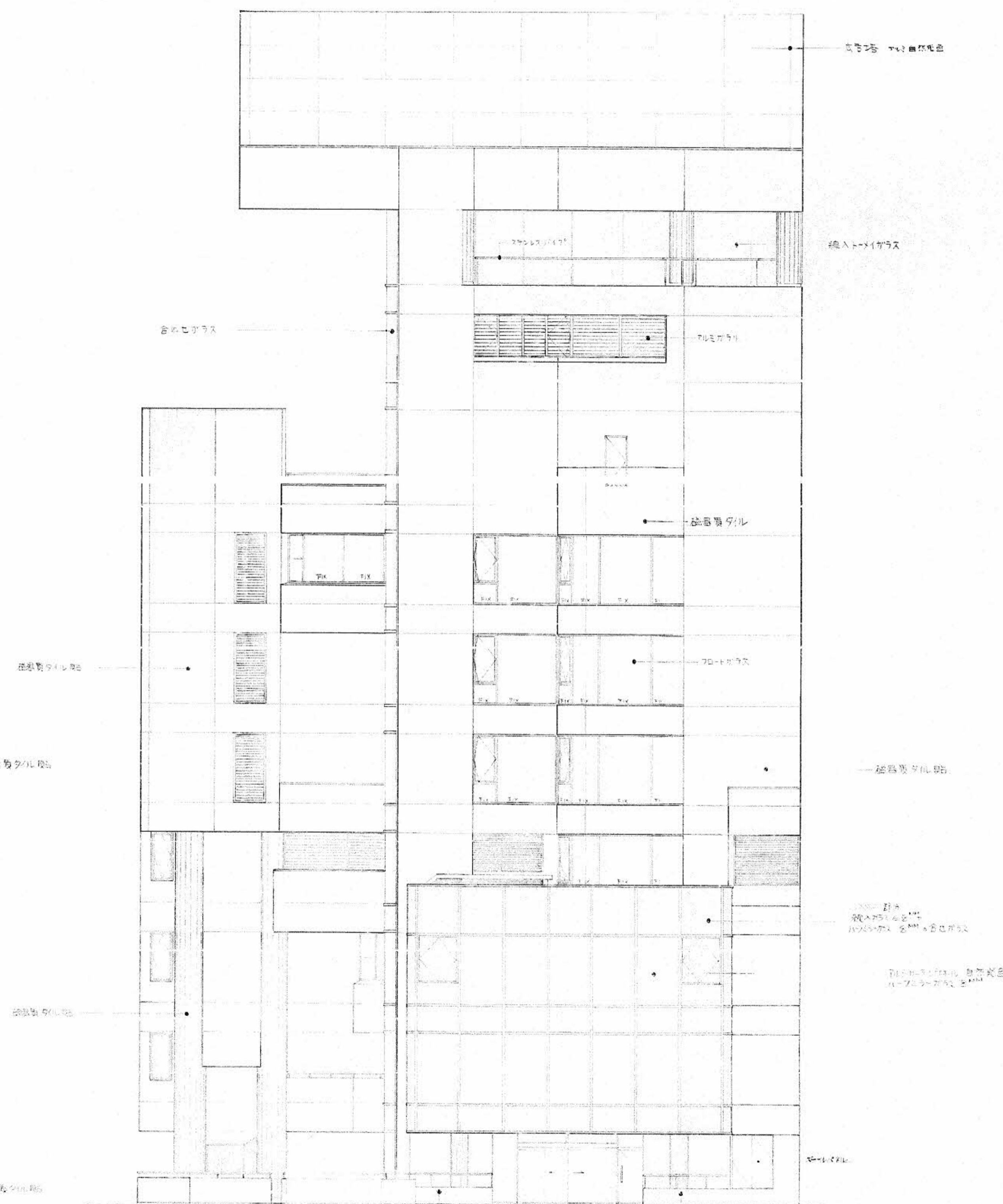
東立面図
