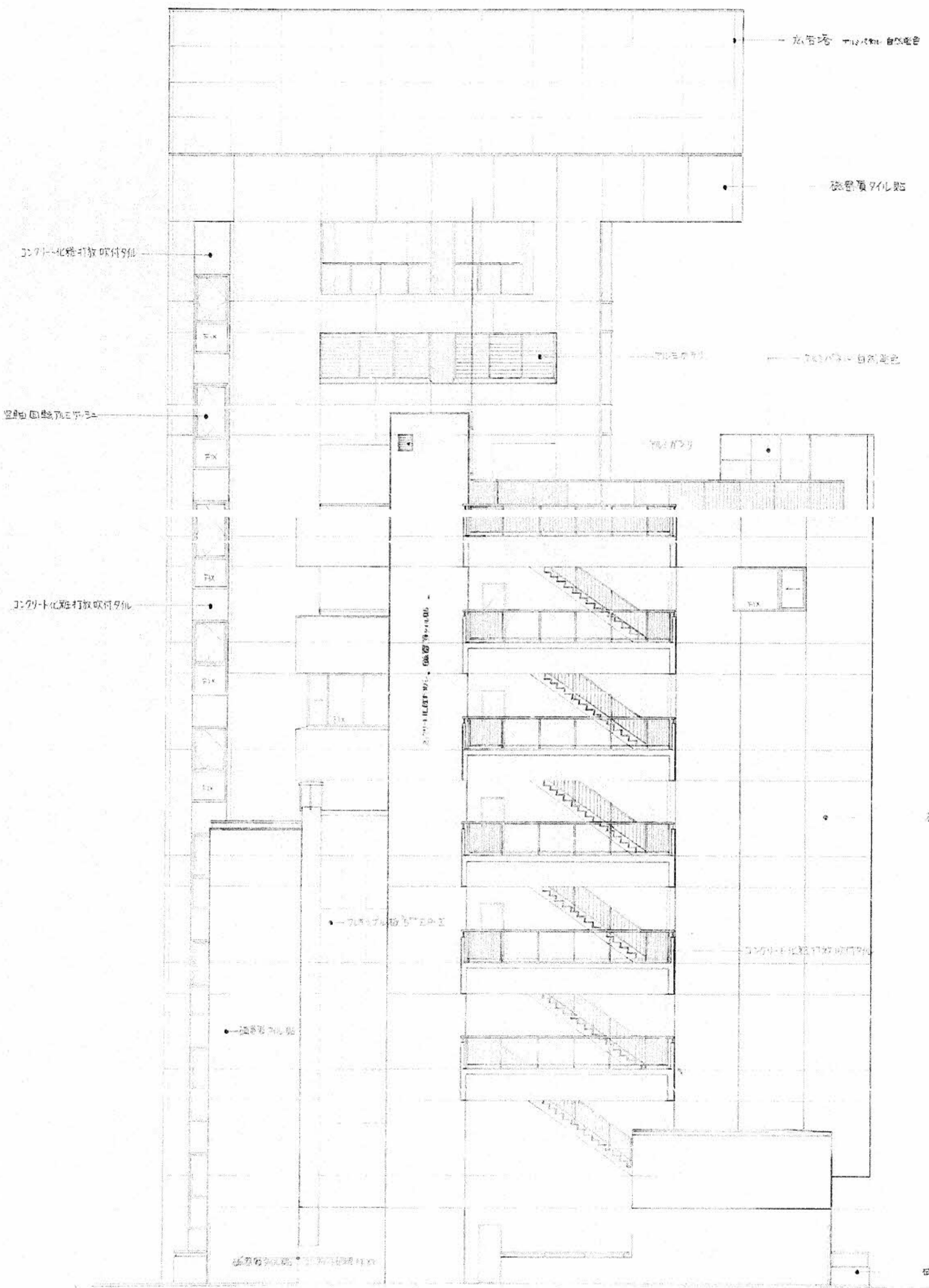
西立面図
