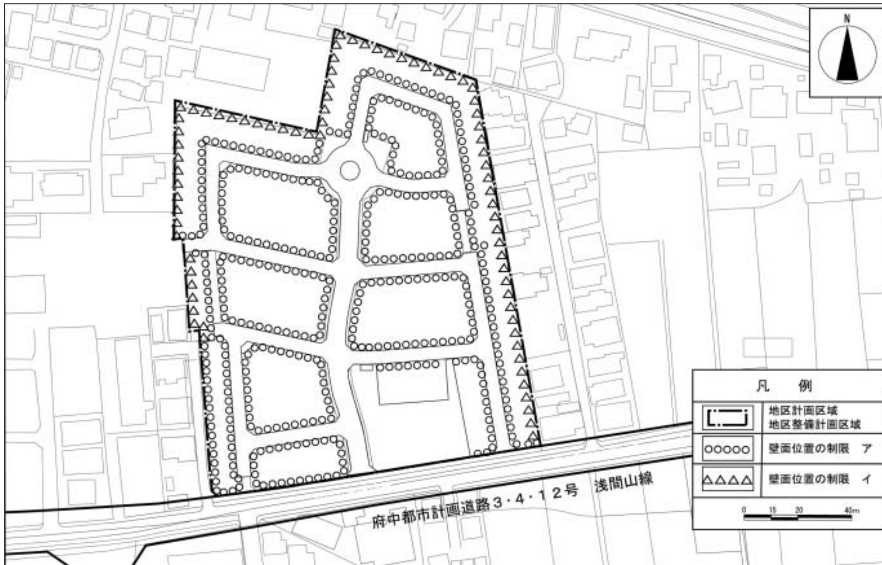
多磨町一丁目住宅地区地区計画 計画図 3
