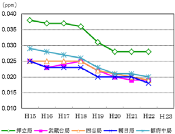
図-二酸化窒素(NO₂)の経年変化
