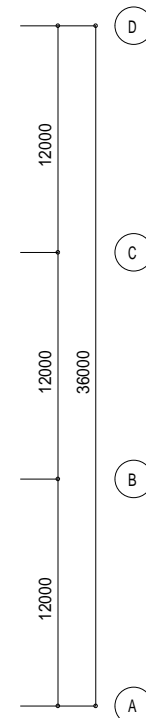
【府中市役所本庁舎】6階平面図
