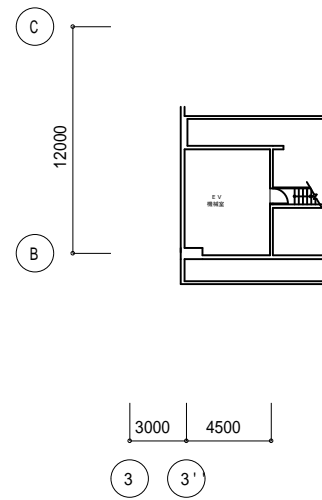
【府中市役所本庁舎】PH1階 (東庁舎) 平面図
