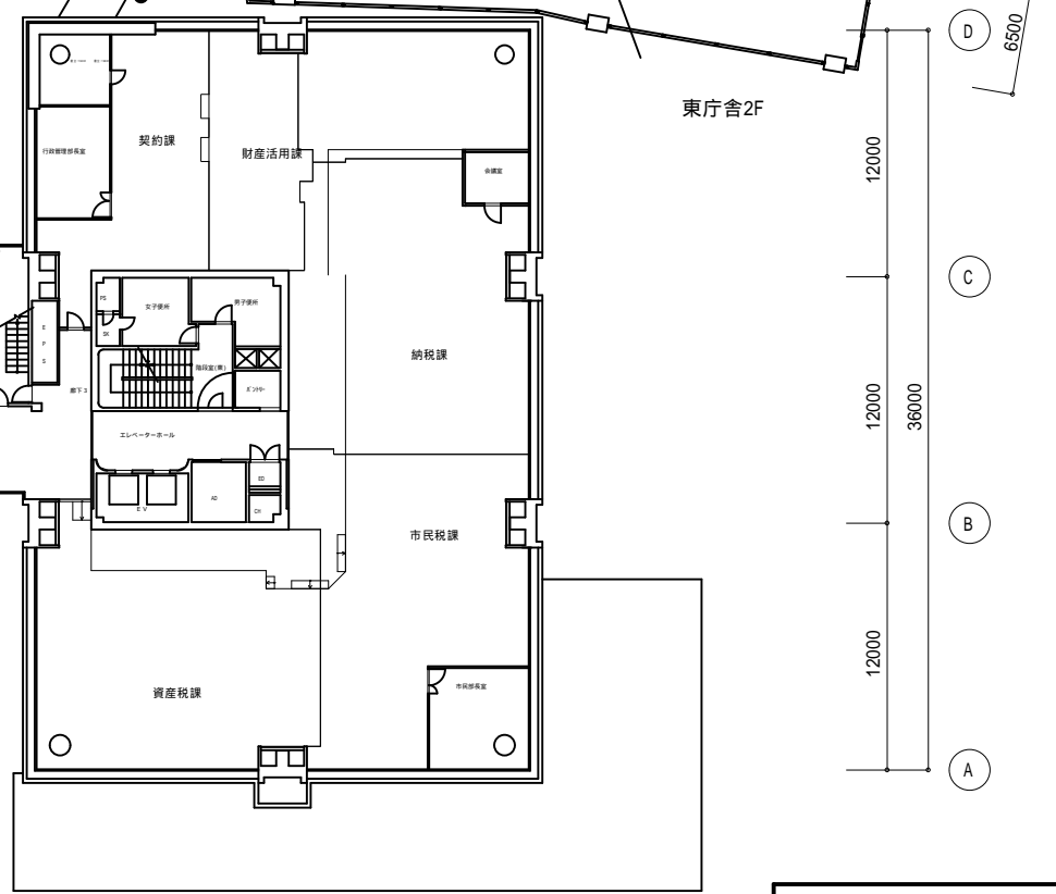
【府中市役所本庁舎】2階平面図
