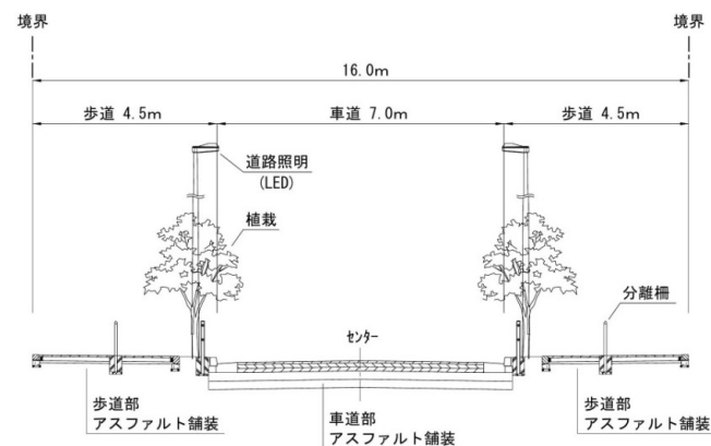
○標準断面図
