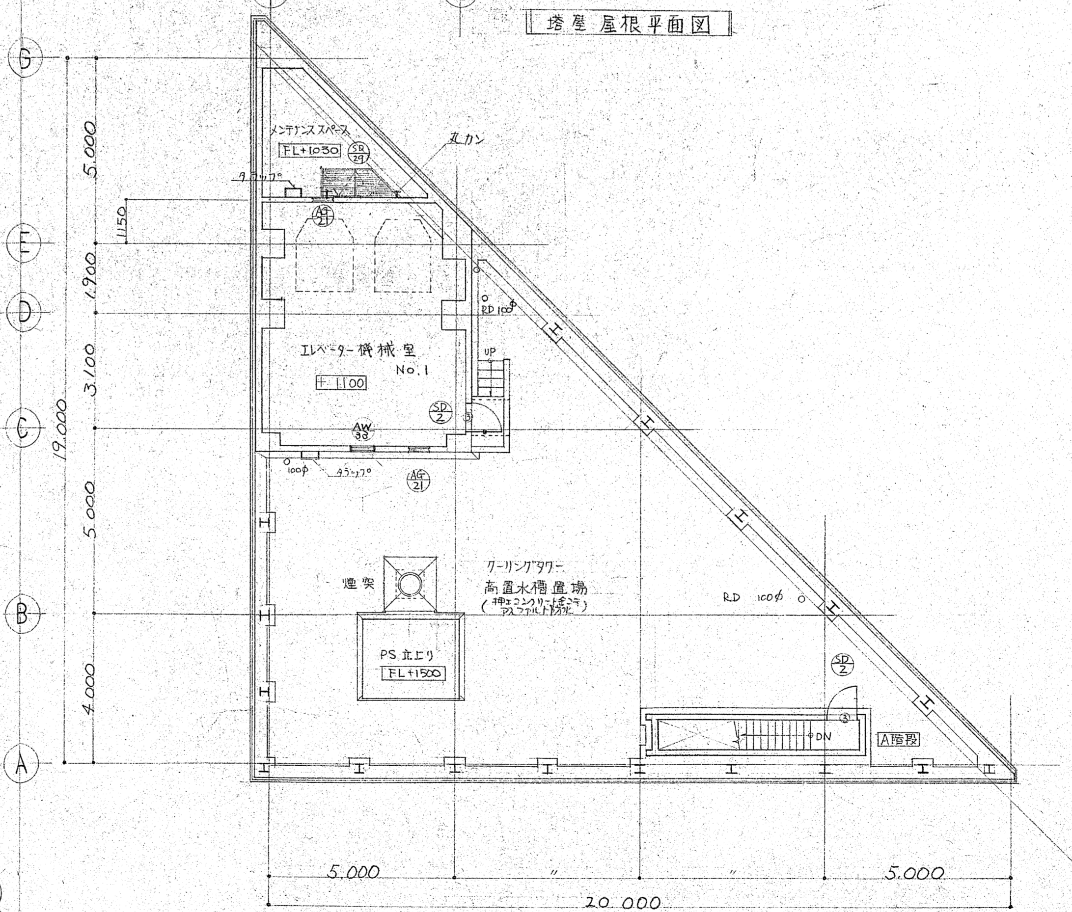
塔屋 3階平面図
