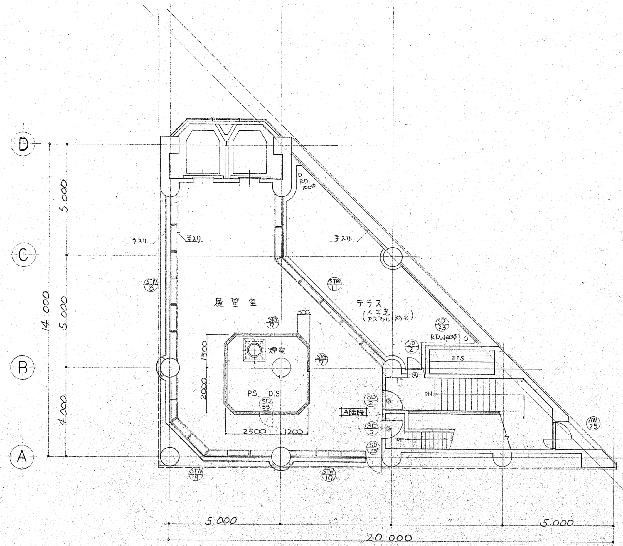
塔屋 2階平面図
