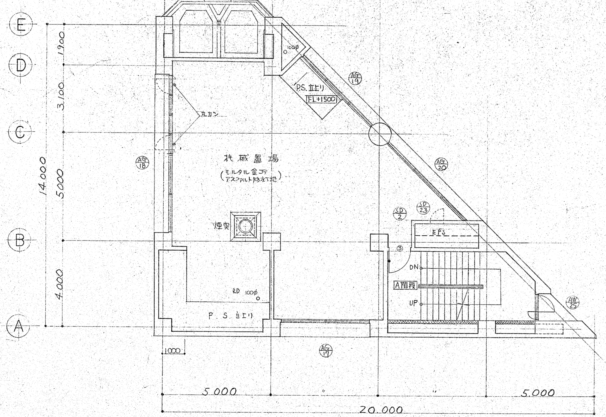
塔屋 2階平面図
