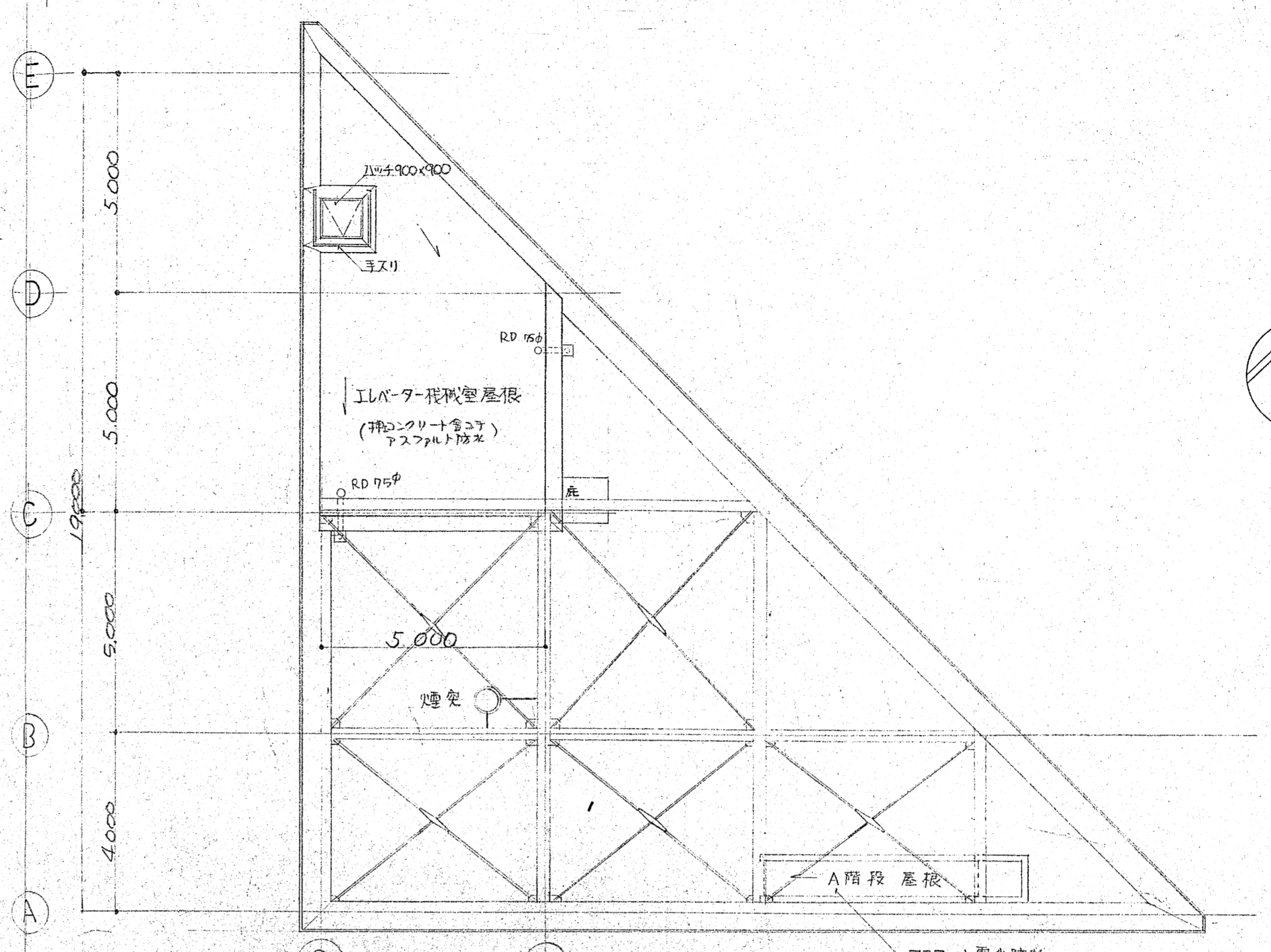
塔屋 屋根平面図
