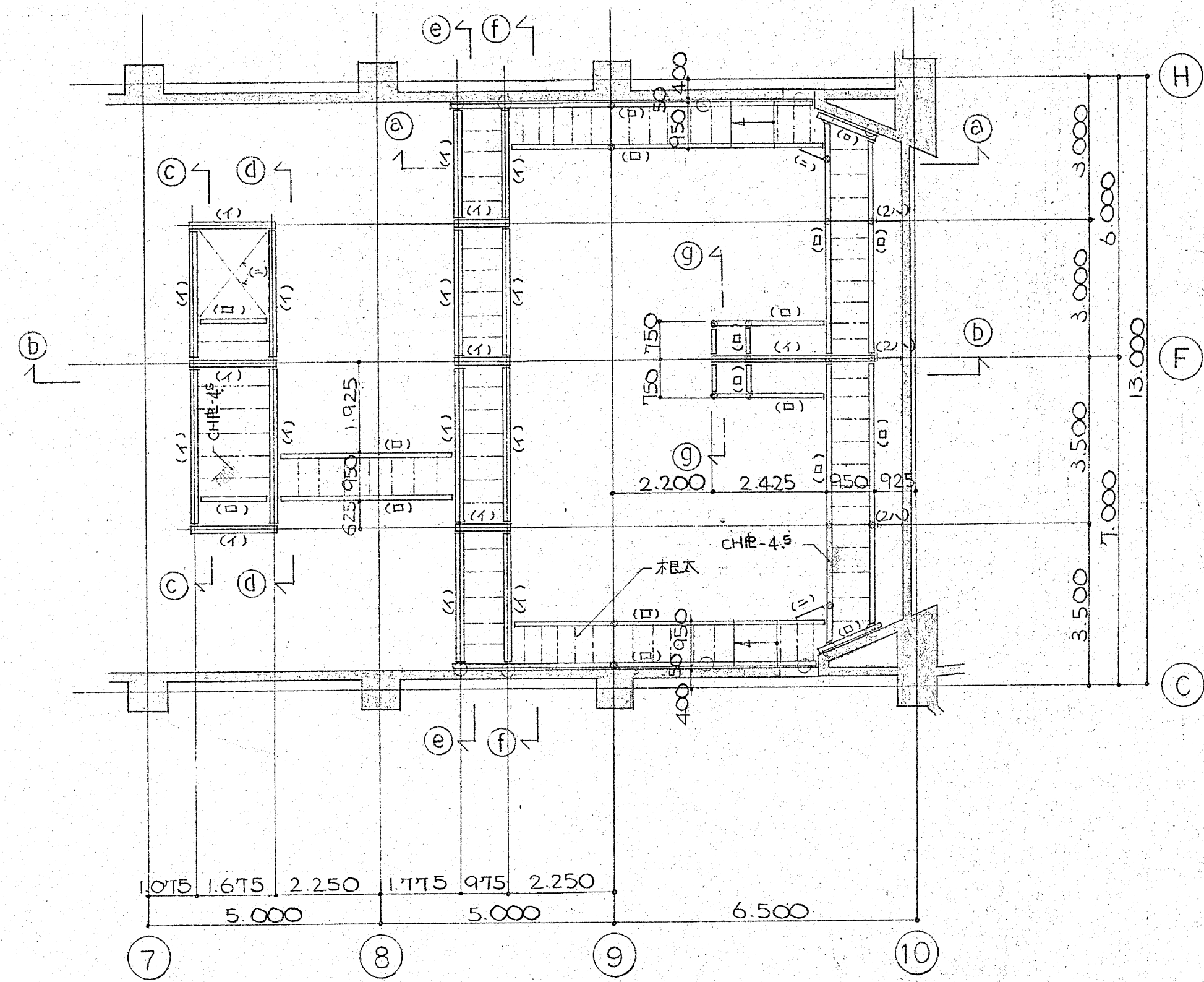
4 階 梁 伏 図 (注1) ●印は 吊点を示し ○印は アンカーボルト 位置を示す。 (吊材は ハとする)
