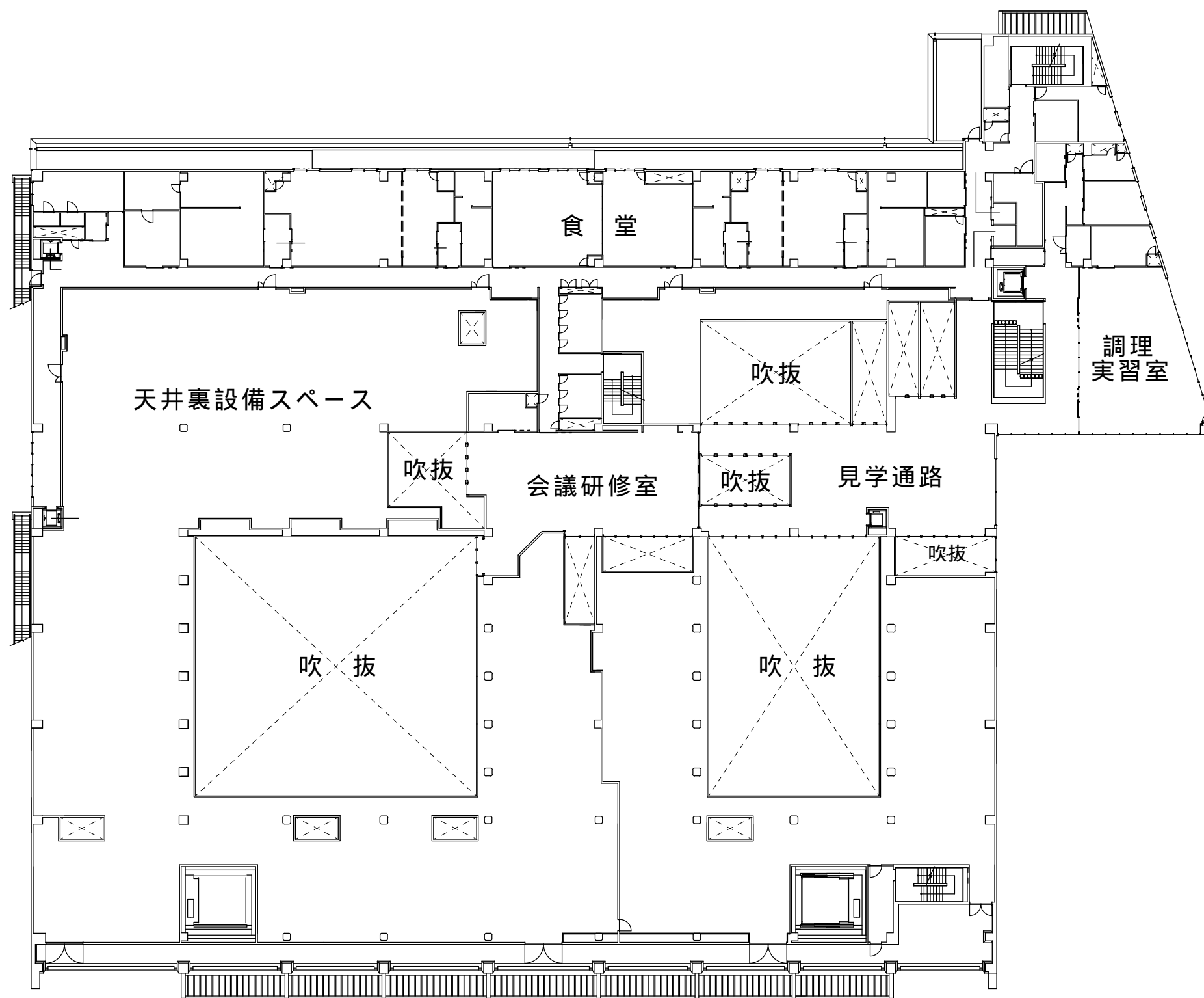
2階平面図
