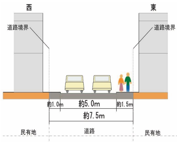
現状の市道4-139号の断面
