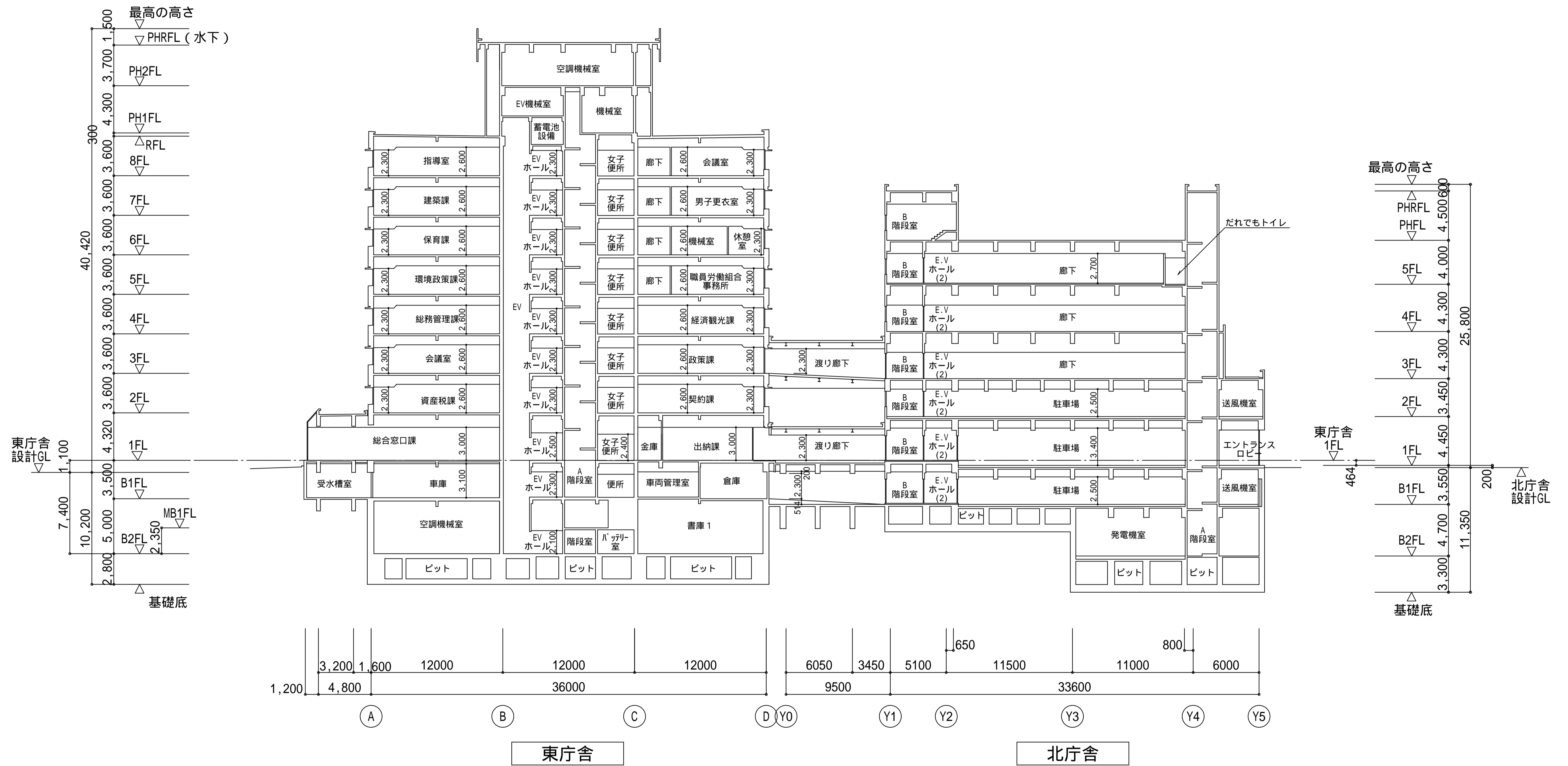
東・北庁舎 断面図
