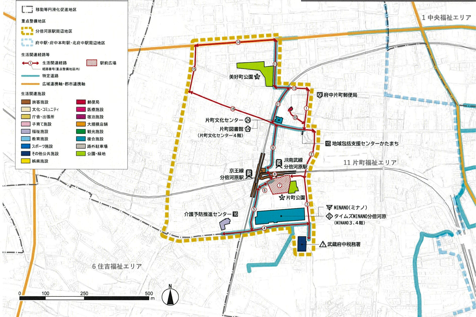
図 分倍河原駅周辺重点整備地区図
