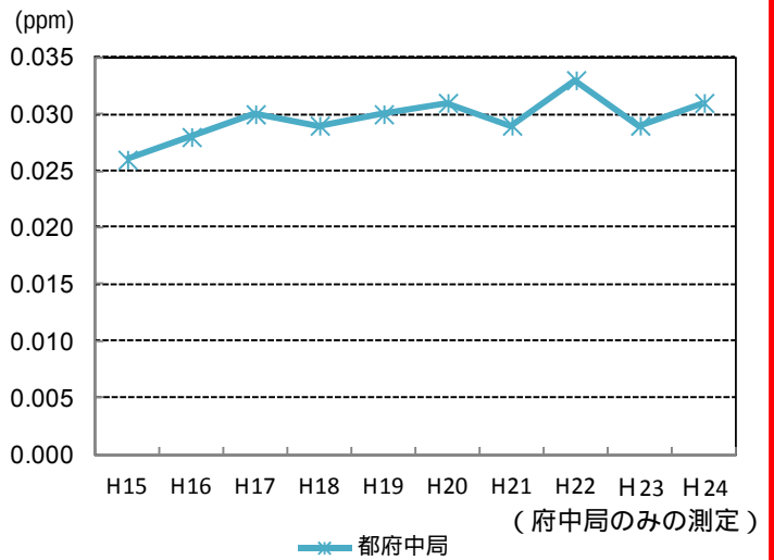
図-オキシダント(Oₓ)の経年変化
