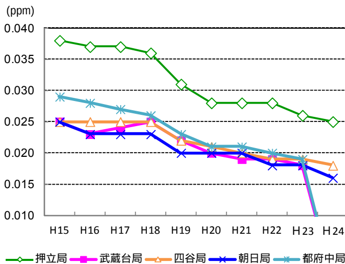
図-二酸化窒素(NO₂)の経年変化
