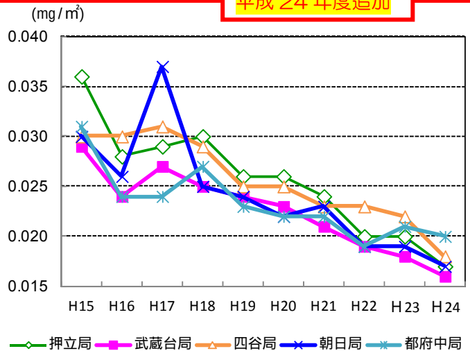
図-浮遊粒子状物質 (SPM) の経年変化
