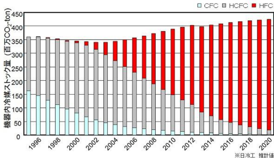
図6 冷凍空調機器の冷媒ストック量
