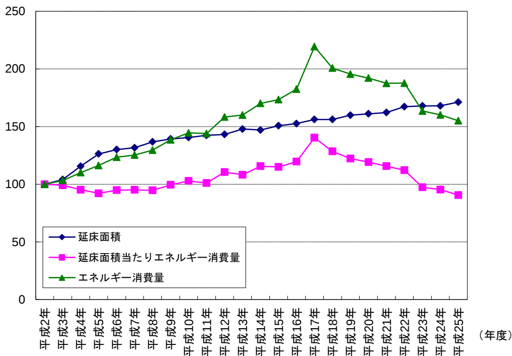
図5 業務部門の床面積あたりのエネルギー消費量
