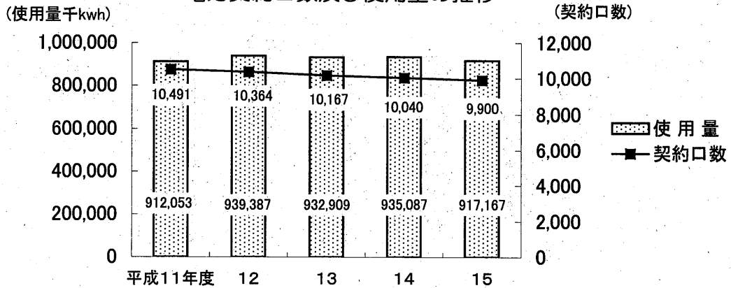
電力契約口数及び使用量の推移
