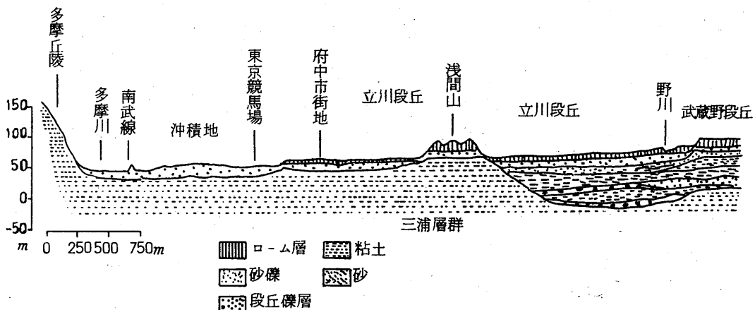
断面図（南北に切る）
