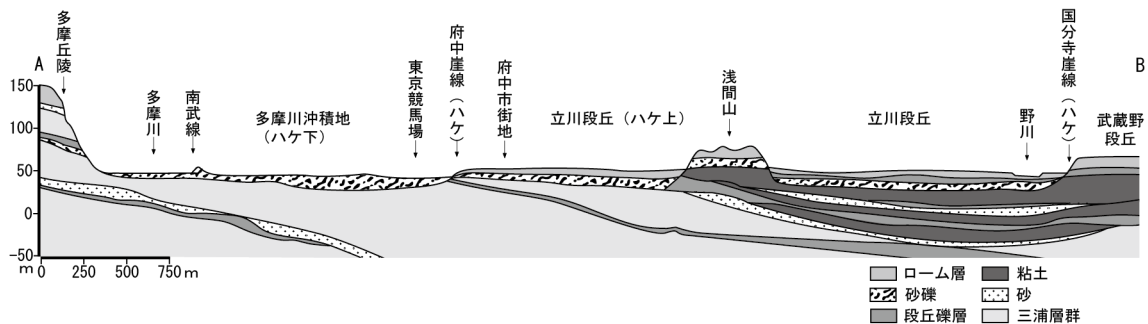
A-B断面模式図
