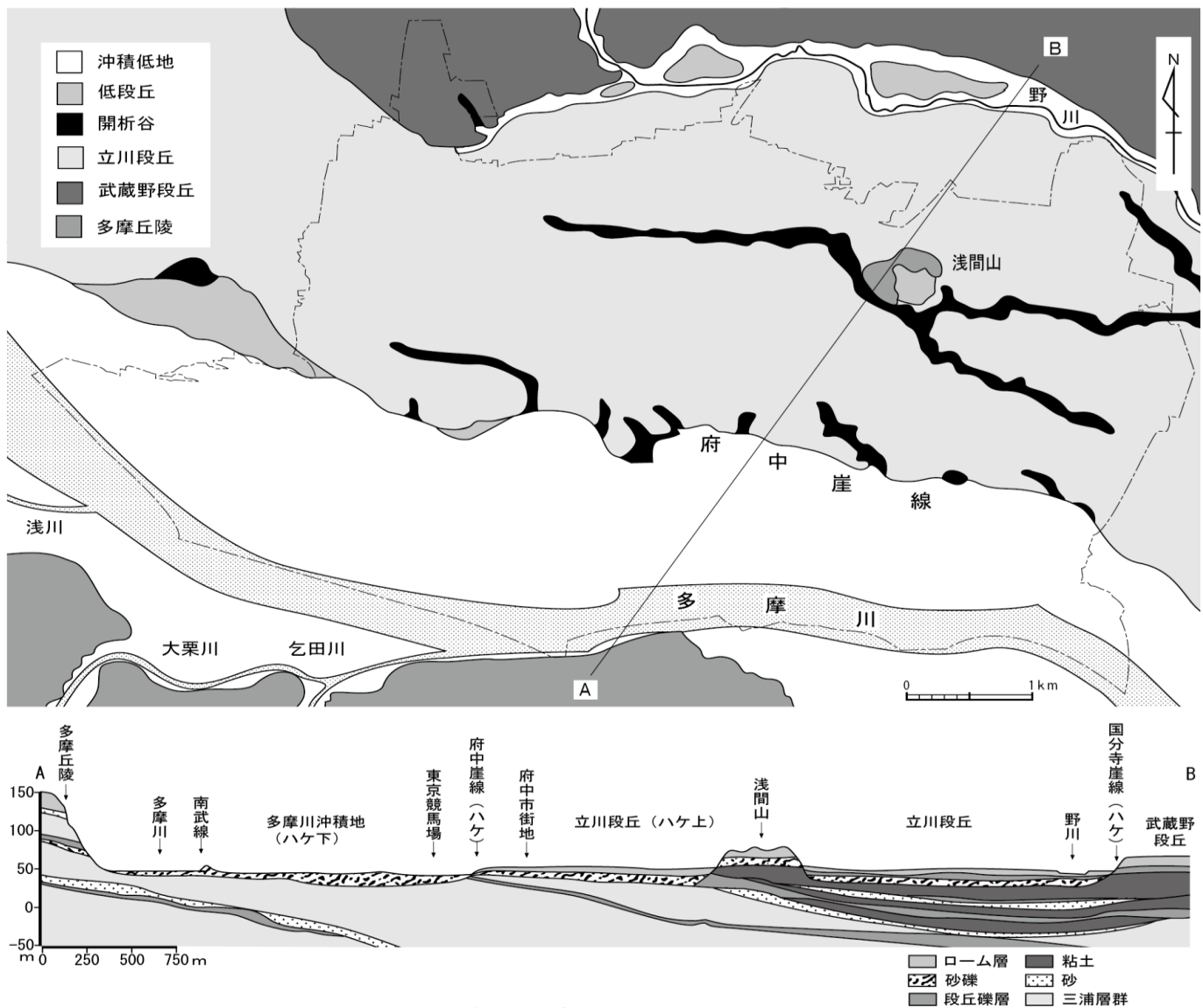
A-B断面模式図
