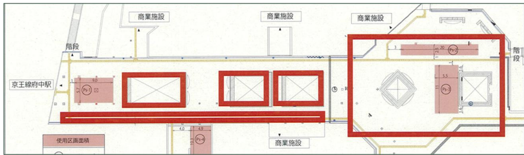
府中駅南口ペデストリアンデッキ配置 詳細
