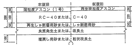
8 車道アスファルト舗装(透水性舗装)
