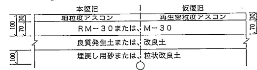
11 歩道アスファルト舗装
