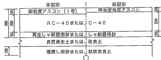
7 車道アスファルト舗装(透水性舗装)
