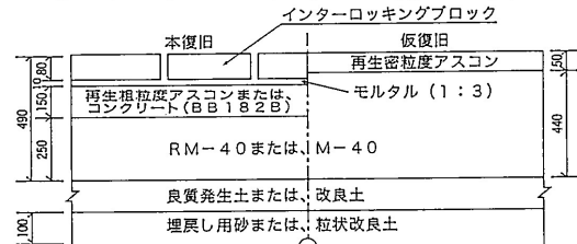
9 インターロッキング舗装 (車道)
