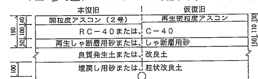
12 歩道アスファルト舗装(透水性舗装)
